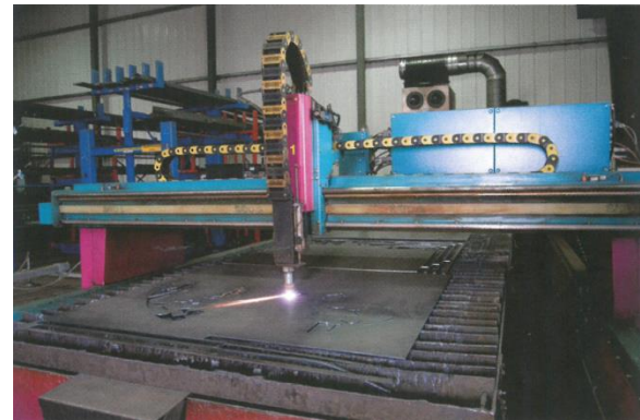
Plasmaschneidanlage 6000x2000mm
